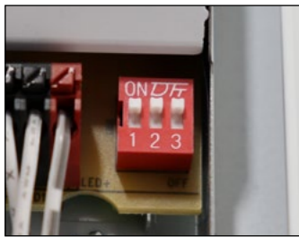
Leistungswahlschalter Power Select switch
