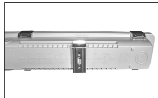
Weit verstellbare Montageclips die man auch zur Seilabhängung nutzen kann Widely adjustable mounting clips that can also be used for suspension ropes
